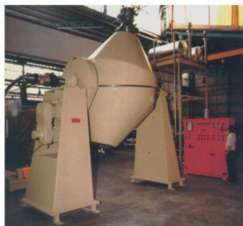
Secador rotativo a vácuo tipo "duplo cone". "Double cone" rotatory vacuum dryer.
